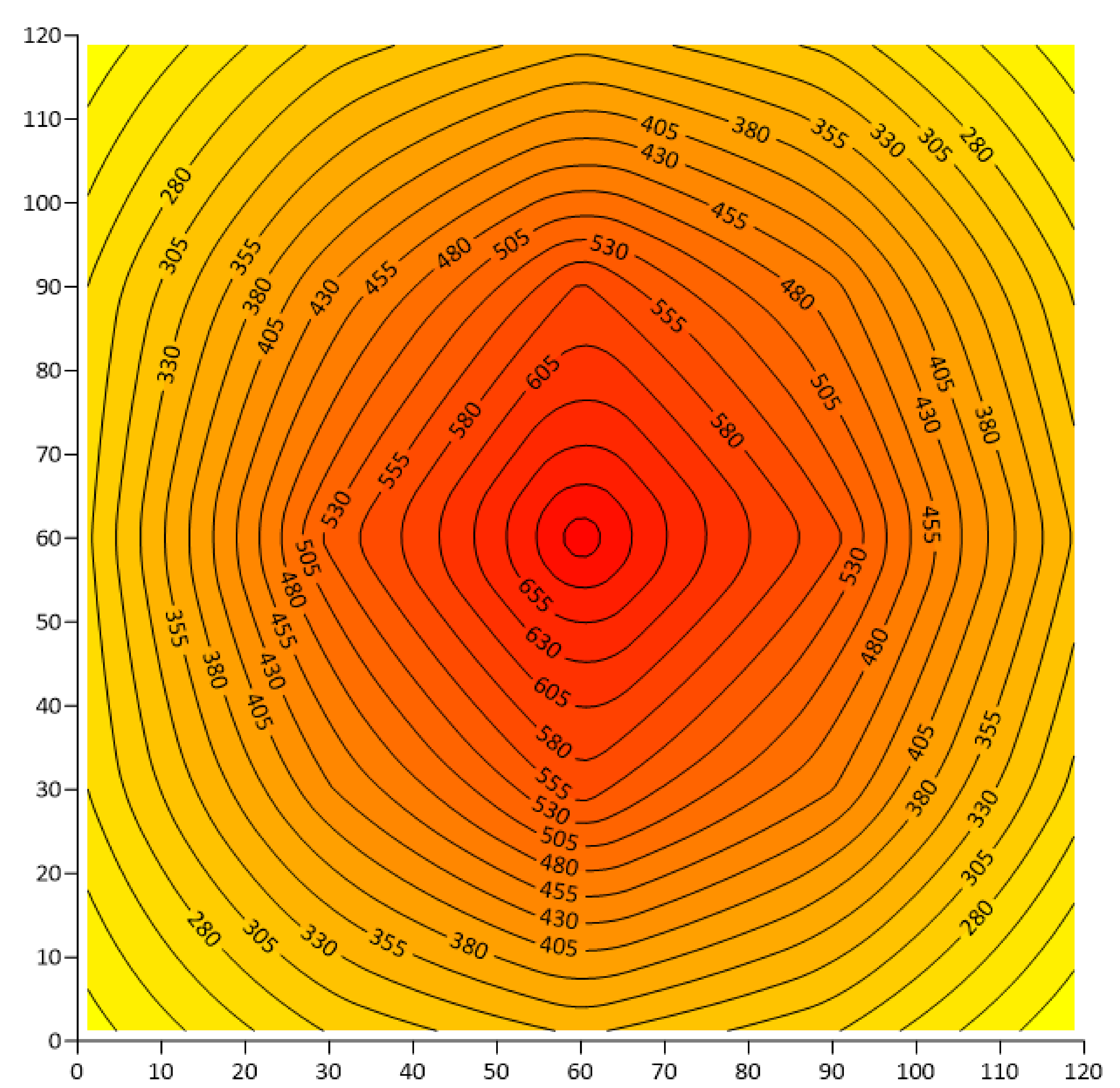
Pro-240W UV + IR a 0,5m
